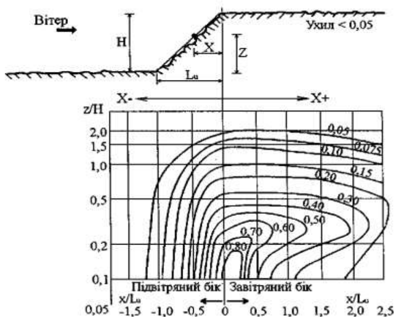
Рисунок 9.3. Коефіцієнт S для схилів
