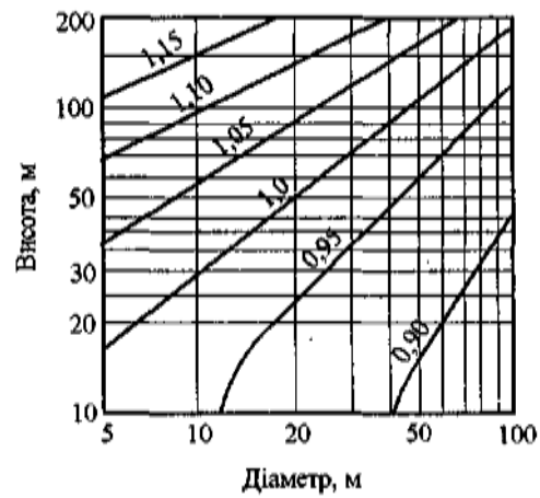
Рисунок 9.6. Коефіцієнт C_d для будівель із сталевим каркасом
