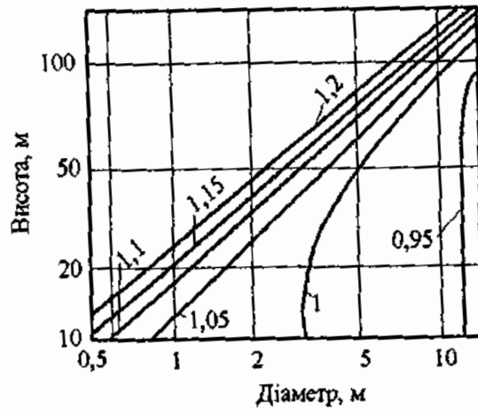
Рисунок 9.9. Коефіцієнт C_d для сталевих труб і апаратів колонного типу з футерівкою
