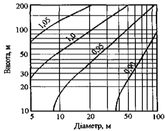
Рисунок 9.7. Коефіцієнт C_d для будівель із сталобетонним каркасом
