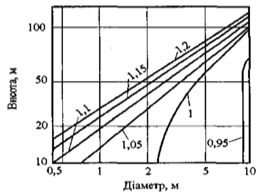
Рисунок 9.8. Коефіцієнт C_d для сталевих труб і апаратів колонного типу без футерівки
