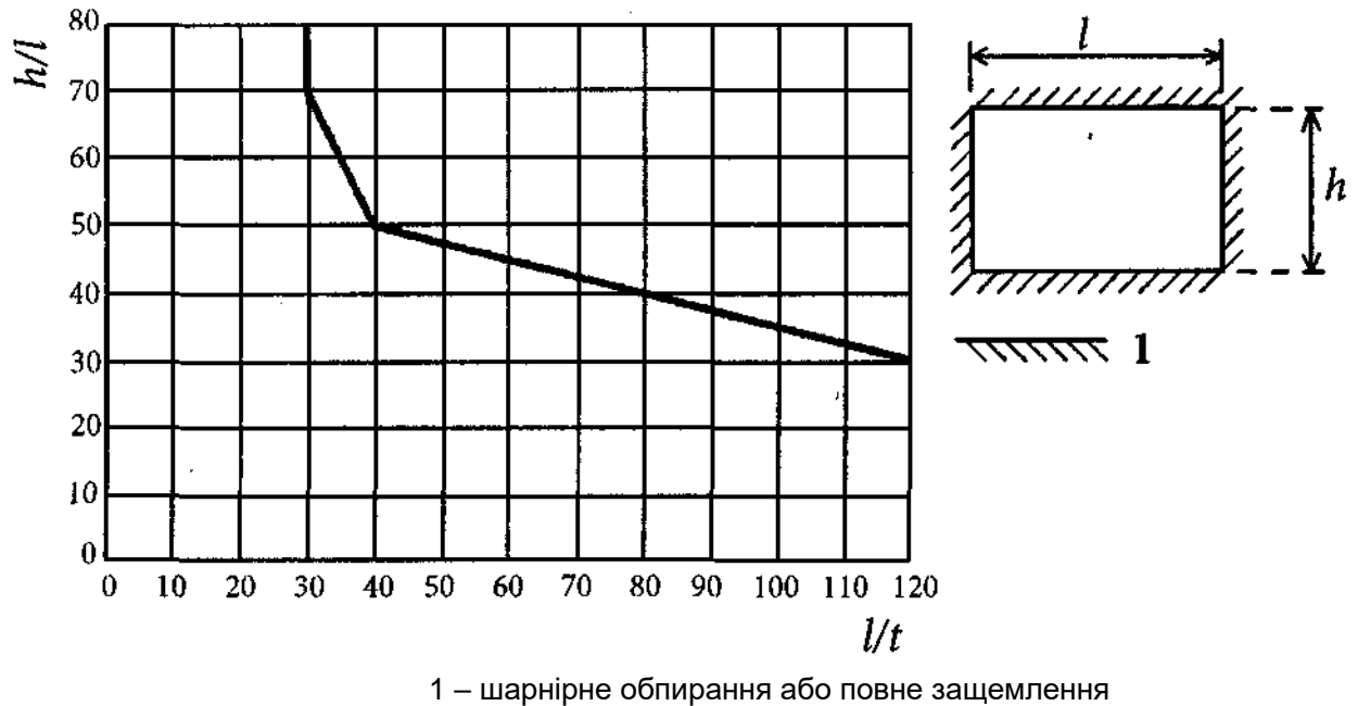
Рисунок И.1 – Граничні відношення висоти і довжини до товщини для стін, закріплених вдовж всіх чотирьох країв
