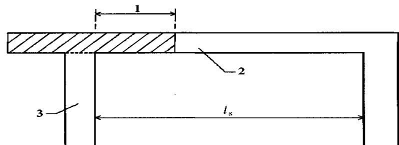
1 – величина, менша за \begin{cases} h_{tot} / 5 \\ l_s / 2 \\ h / 2 \\ 6 t \end{cases} ; 2 – перетинаюча стіна; 3 – стіна-діафрагма
