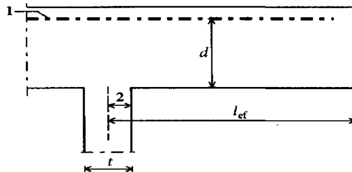
1 - арматура; 2 - t/2 або d/2 залежно від того, яке значення менше
