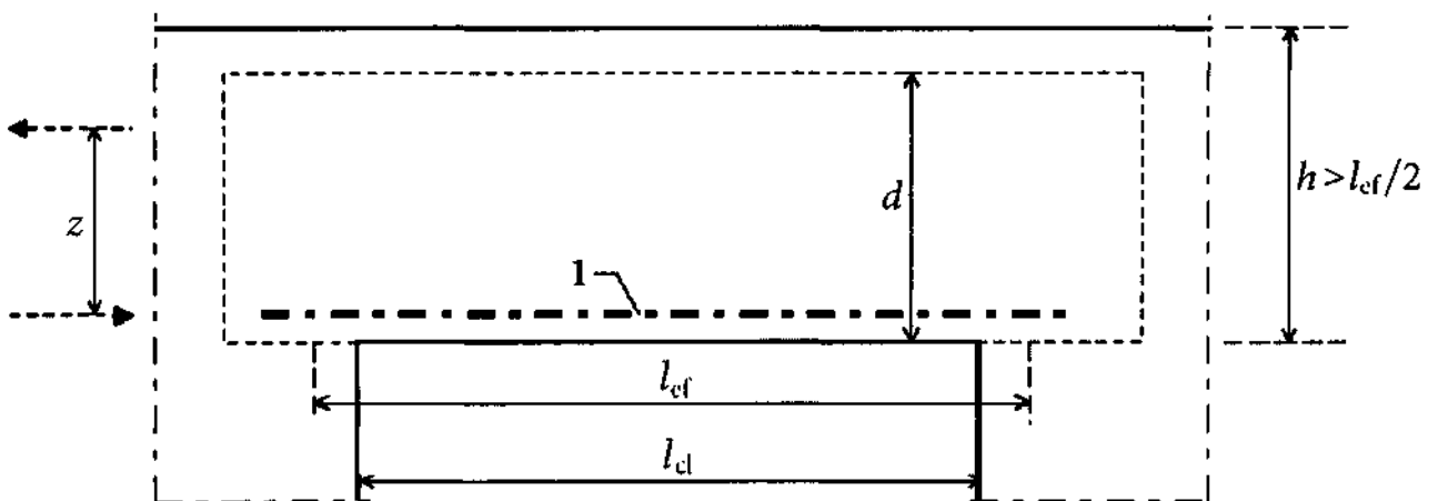
Рисунок 11.7 – Арматура балки-стілки
