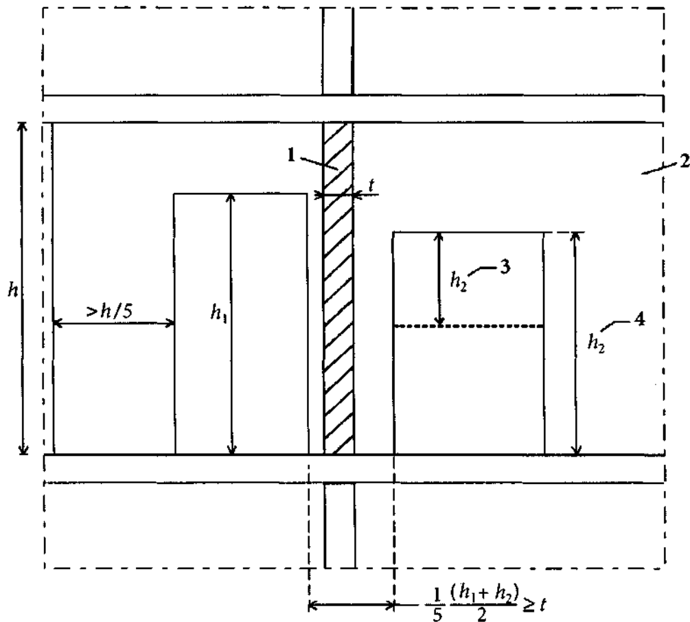
Рисунок 10.1 – Мінімальна довжина діафрагми жорсткості з отворами
