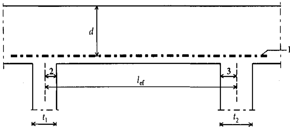
1 - арматура; 2 - t_1/2 або d/2 залежно від того, яка величина менша; 3 - t_2/2 або d/2 залежно від того, яка величина менша
