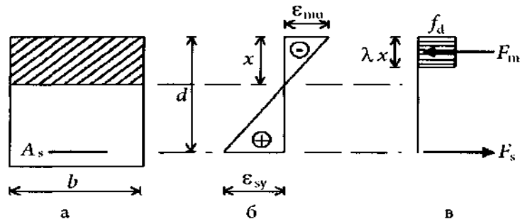
а – поперечний переріз; б – деформації; в – внутрішні сили
