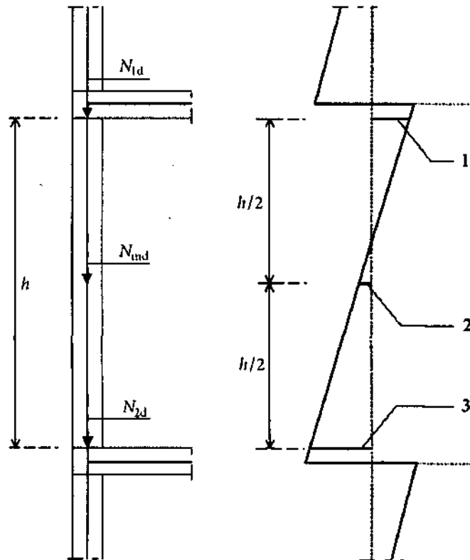
1 – M_{1d} (на нижній стороні перекриття); 2 – M_{md} (на середині висоти стіни); 3 – M_{2d} (зверху перекриття) Рисунок 11.1 – Моменти внаслідок ексцентриситету
