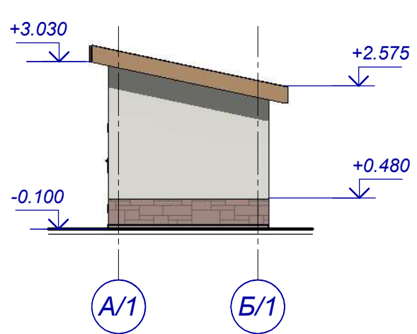
Боковий фасад 1:100
