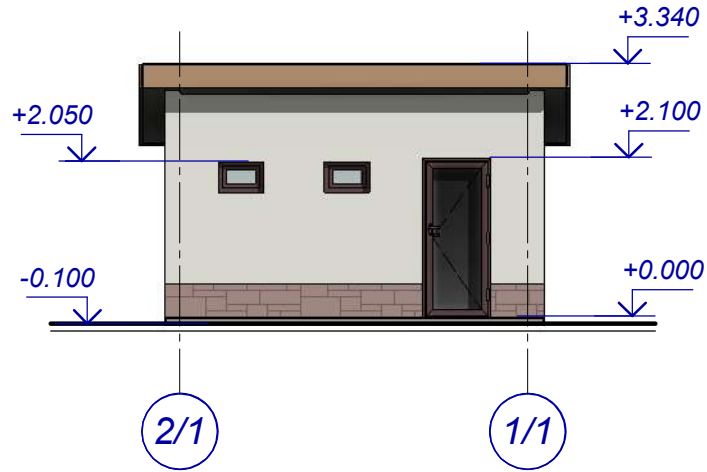
Головний фасад 1:100
