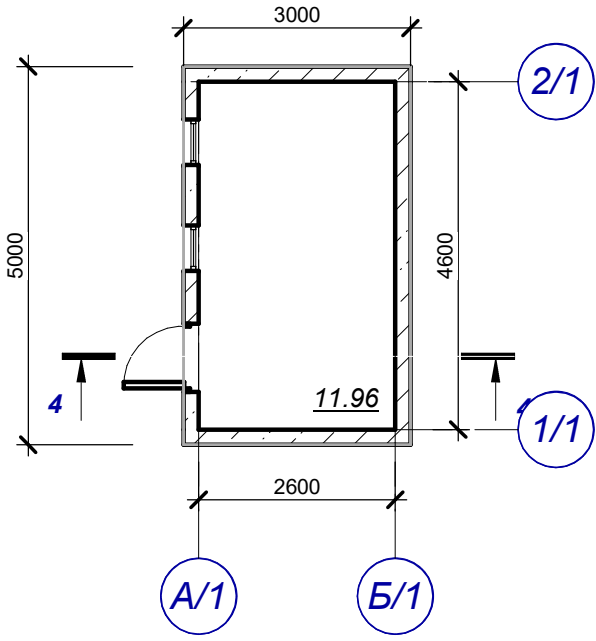
План на відм. 0,000 1:100
