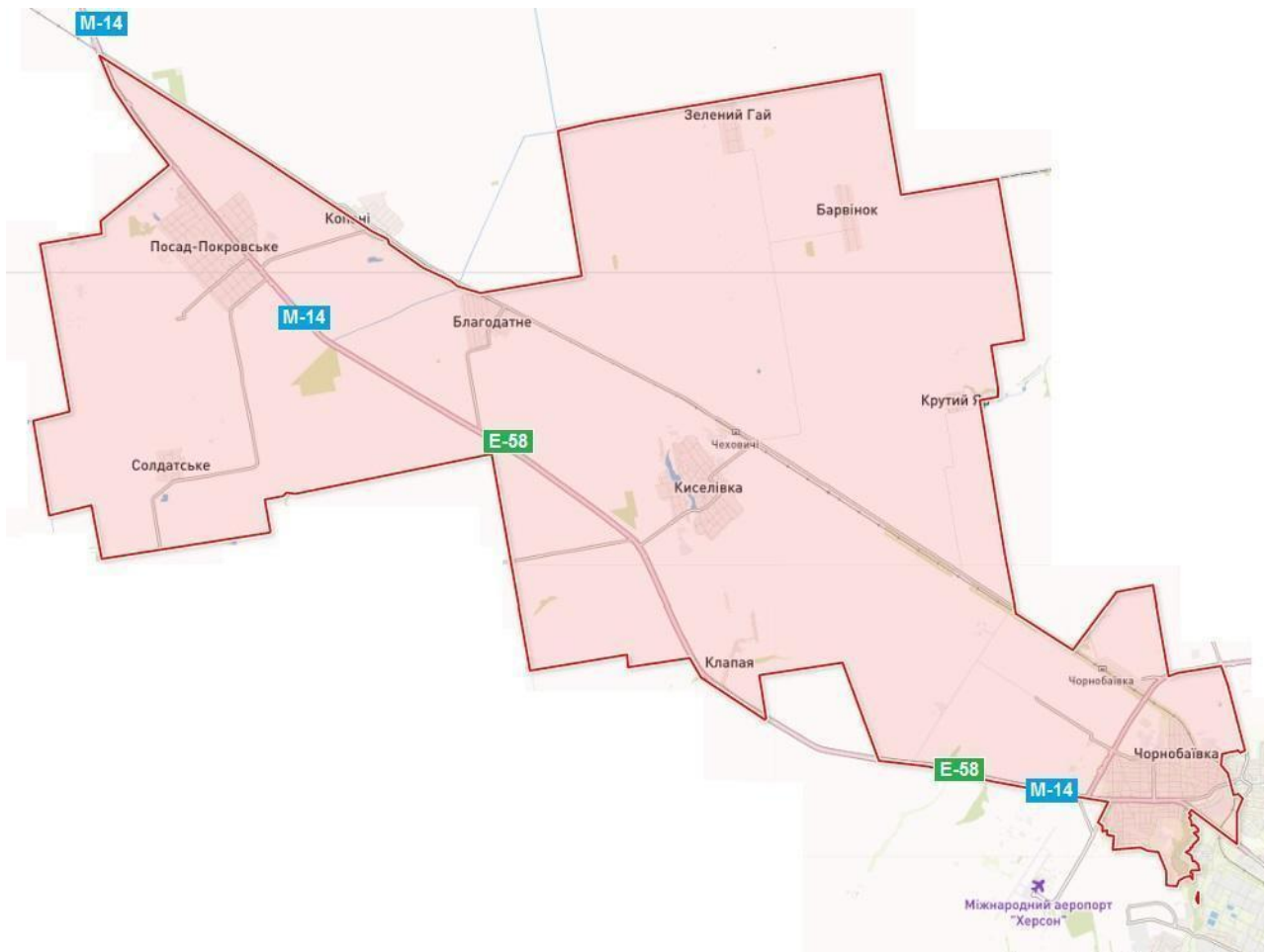
Рисунок 1.3 – Транспортна мережа на території Чорнобаївської ТГ 7
