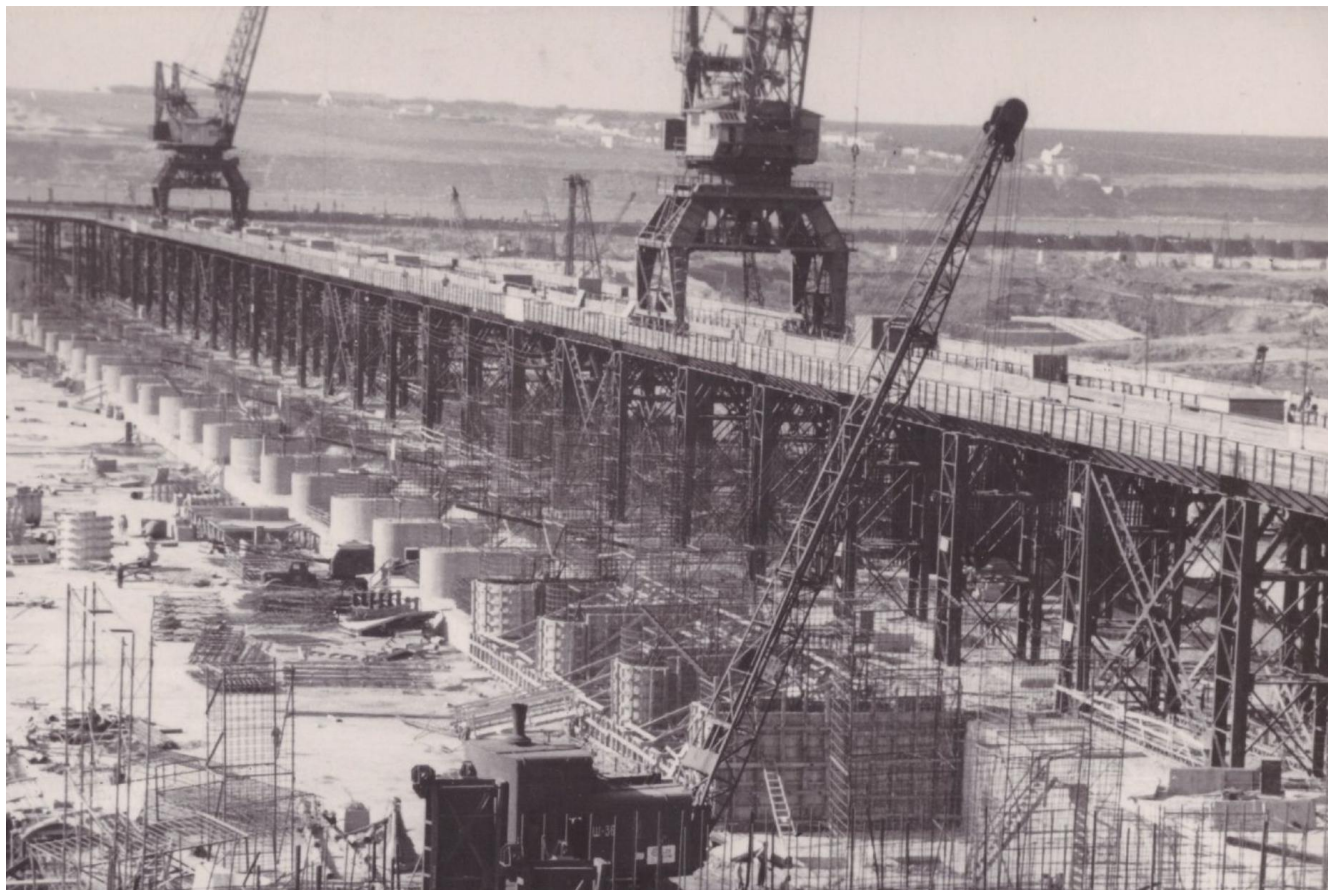
Рисунок 1.4 – Будівництво Каховської ГЕС
