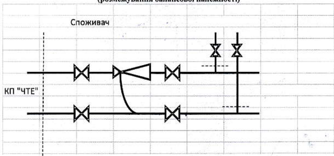
Схема межі експлуатаційної відповідальності сторін (розмежування балансової належності)
