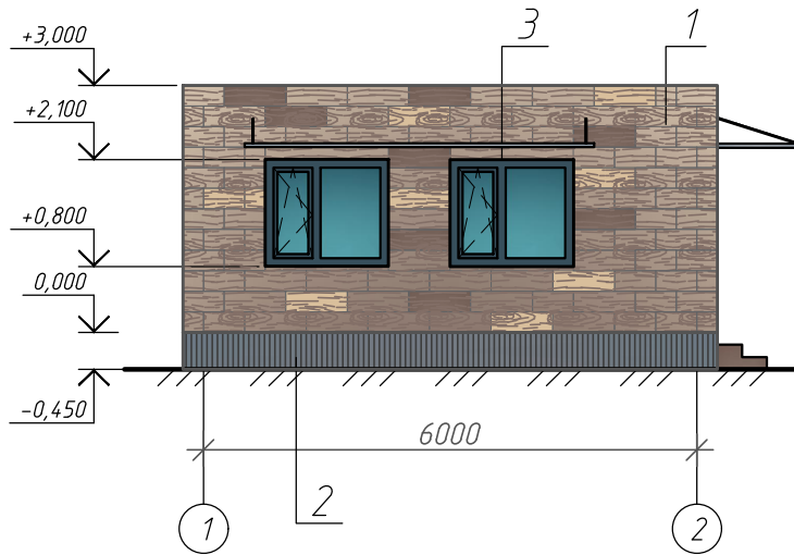
Фасад 1-2
