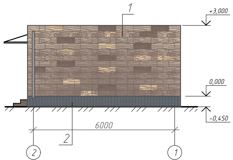
Фасад 2-1
