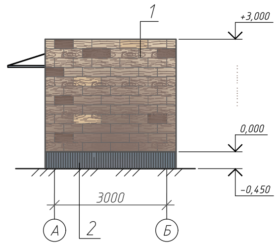
Фасад Б-А
