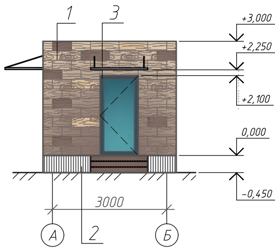
Фасад А-Б
