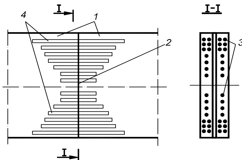
Рис. 6.1 Клеєштирьовий стик
