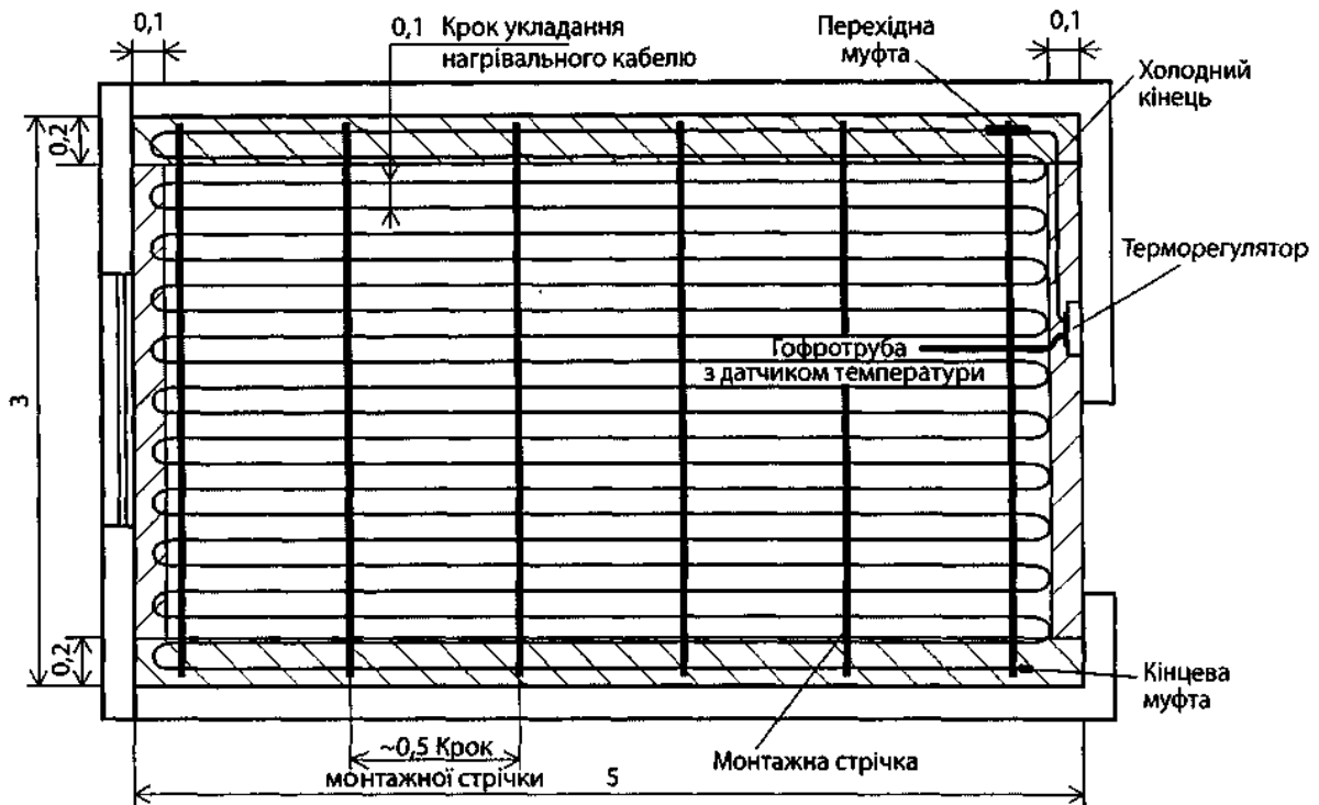
Рисунок В.3 - Варіант розташування елементів ЕКС ОПД В.2.16 Розріз підлоги з нагрівальним кабелем показано на рисунку В.4.
