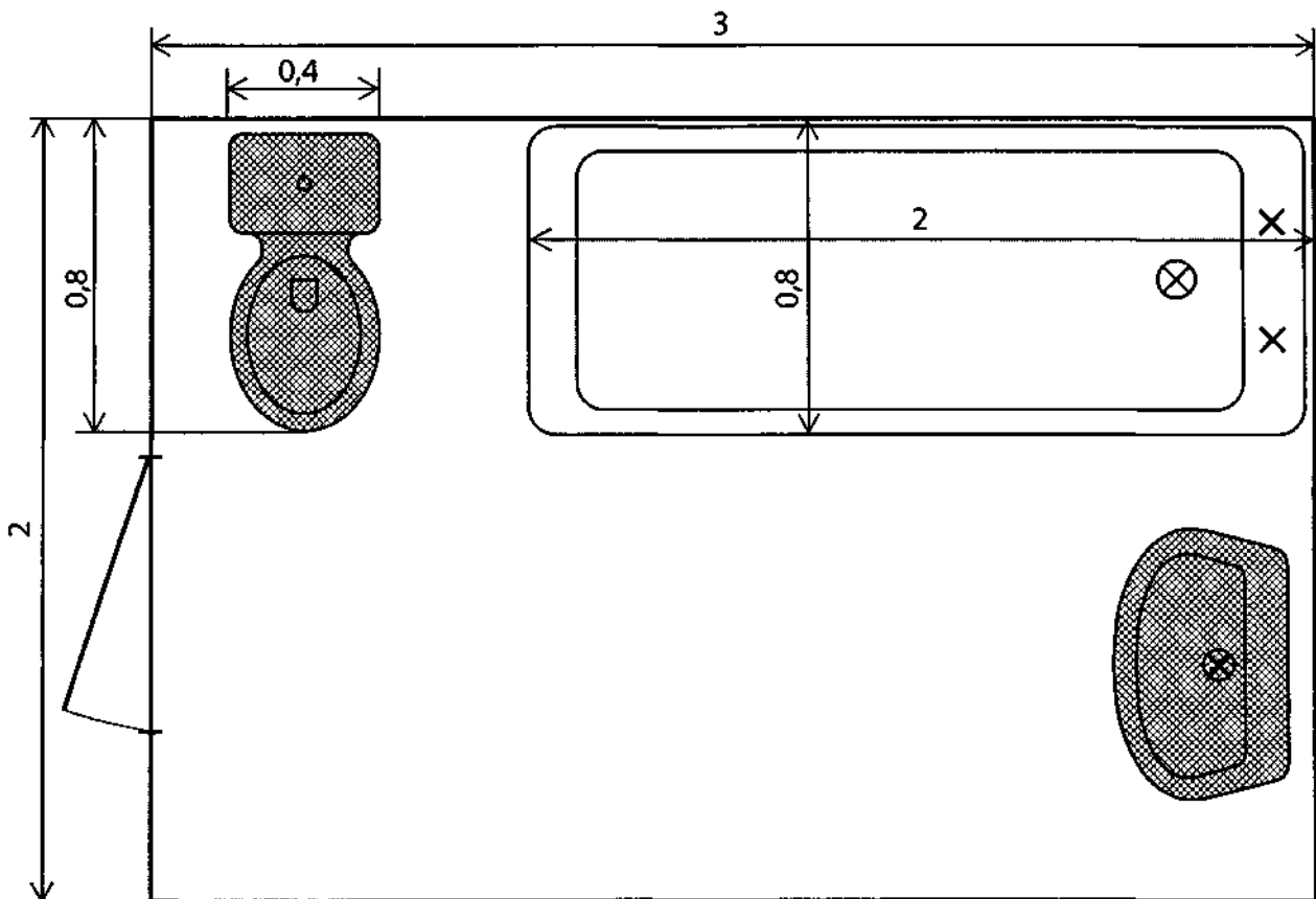
Рисунок А.1 - План суміщеного санвузла
