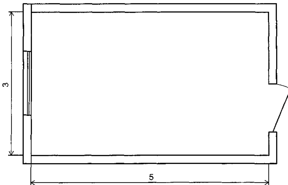
Рисунок В.1 - План житлової кімнати Шари
