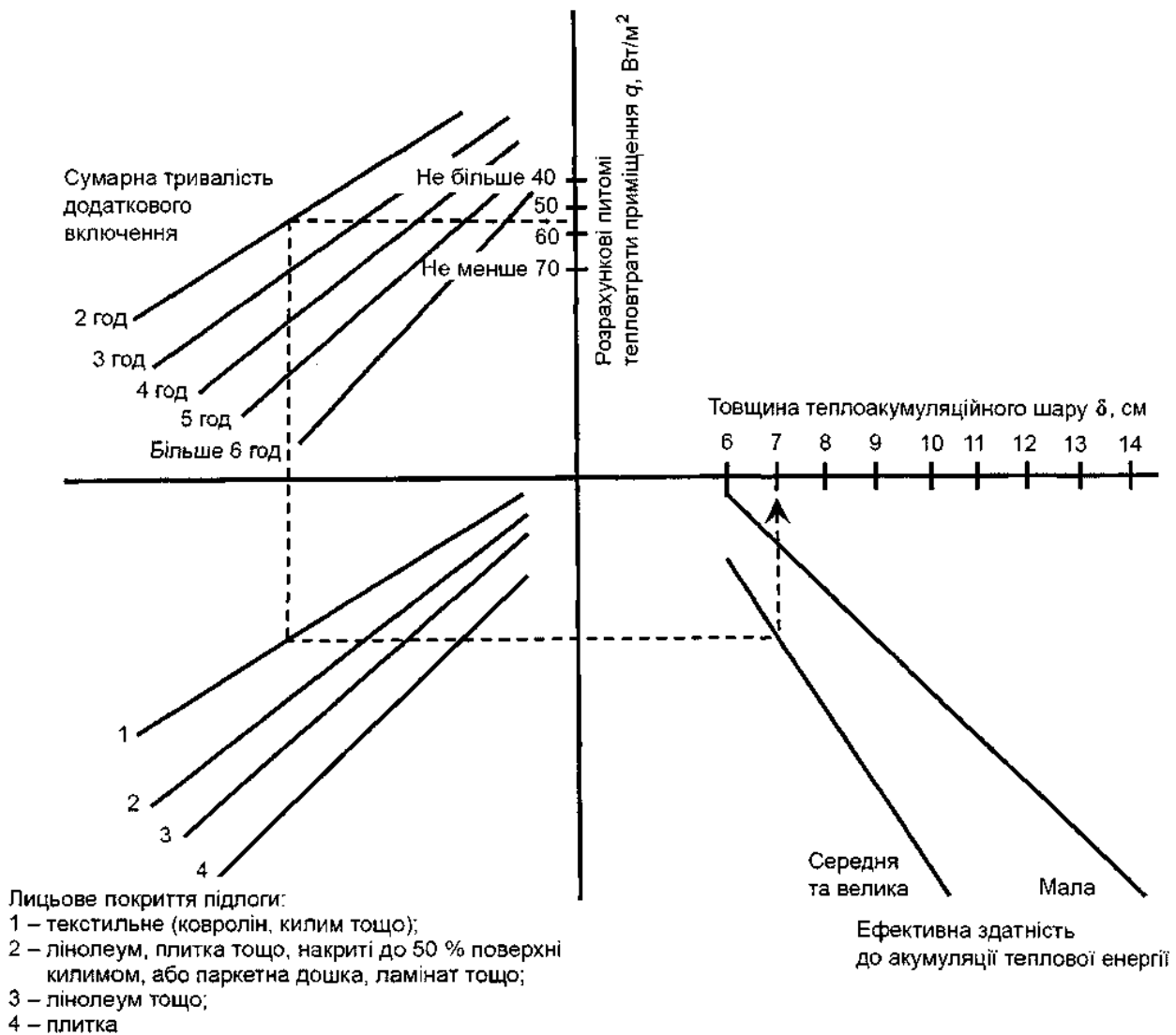
Рисунок 2 - Номограма з визначення товщини теплоакумуляційного шару ЕКС ОТА
