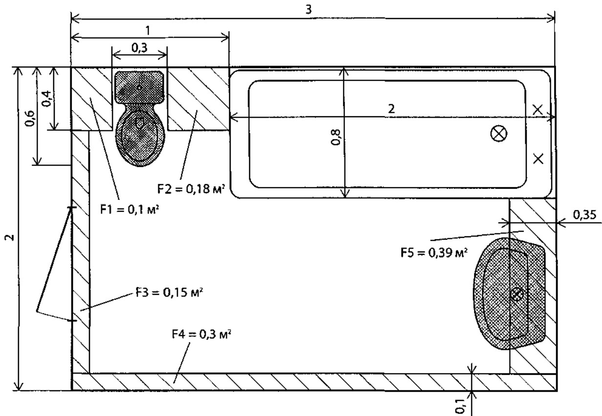
Рисунок А.2 - Визначення зон, у яких не встановлюють нагрівальний кабель. За рисунком А.2 площа виділених зон становить:
