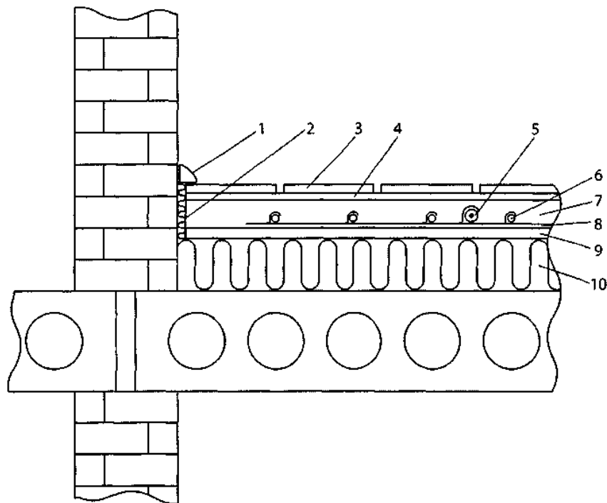
1 - плінтус; 2 - торцева деформаційна стрічка; 3 - лицьове покриття, паркетна дошка; 4 - розділювальний шар під паркетну дошку; 5 - датчик температури підлоги в захисній трубці; 6 - нагрівальний кабель; 7 - суцільний шар над нагрівальним кабелем (цементно-піщана стяжка); 8 - монтажна стрічка; 9 - цементно-піщана стяжка під нагрівальним кабелем; 10 - теплоізоляція
