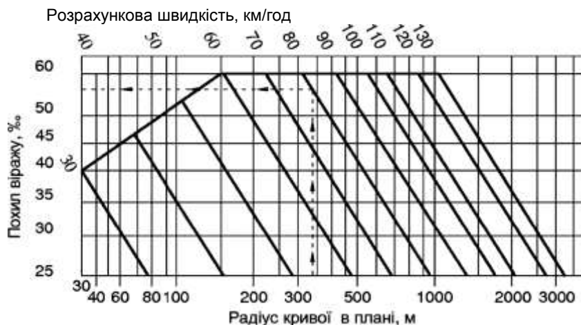
Рисунок 5.1 - Номограма для визначення похилу віражу
