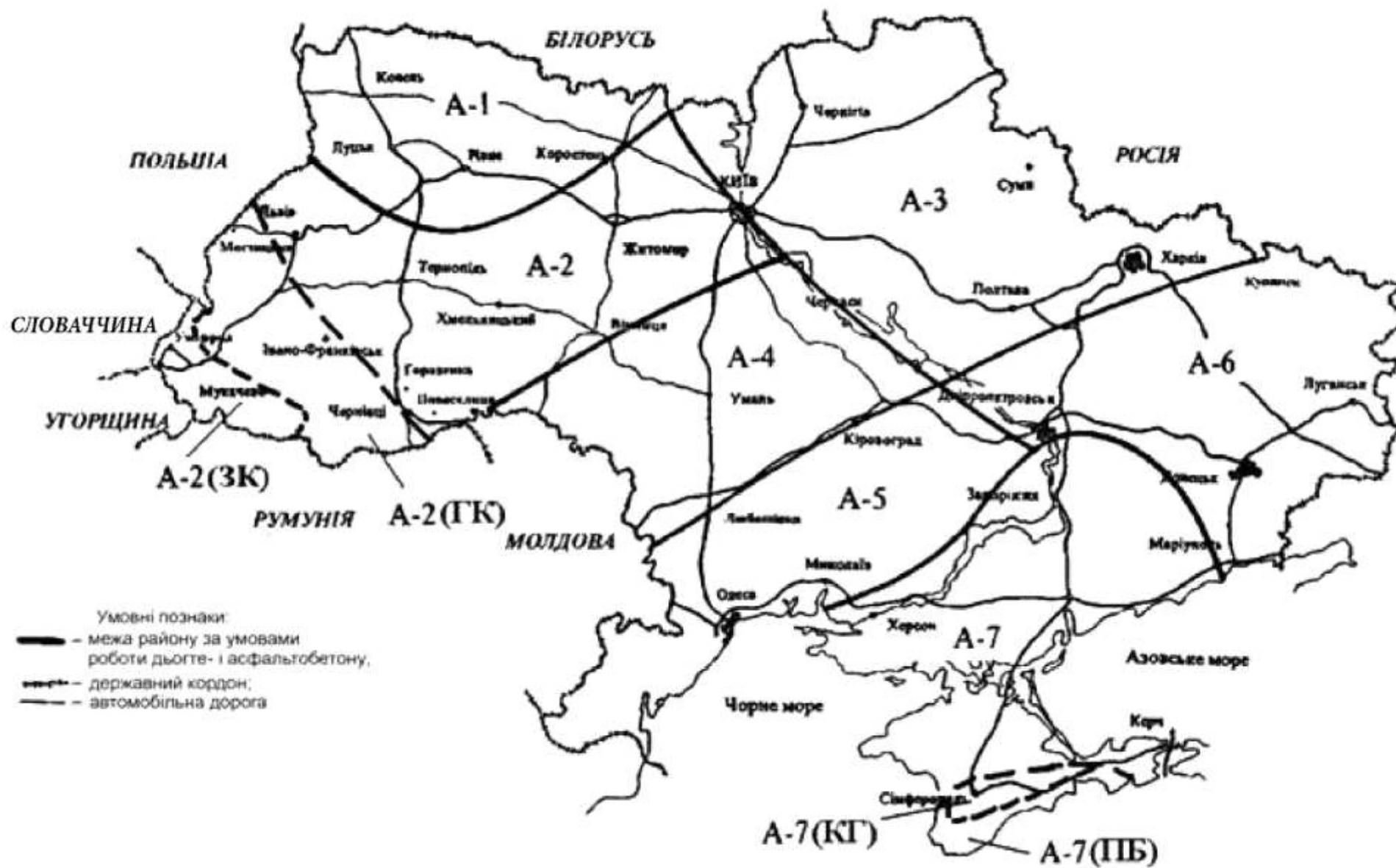
Рисунок Д - Районування території України за кліматичними умовами роботи асфальтобетонного покриття
