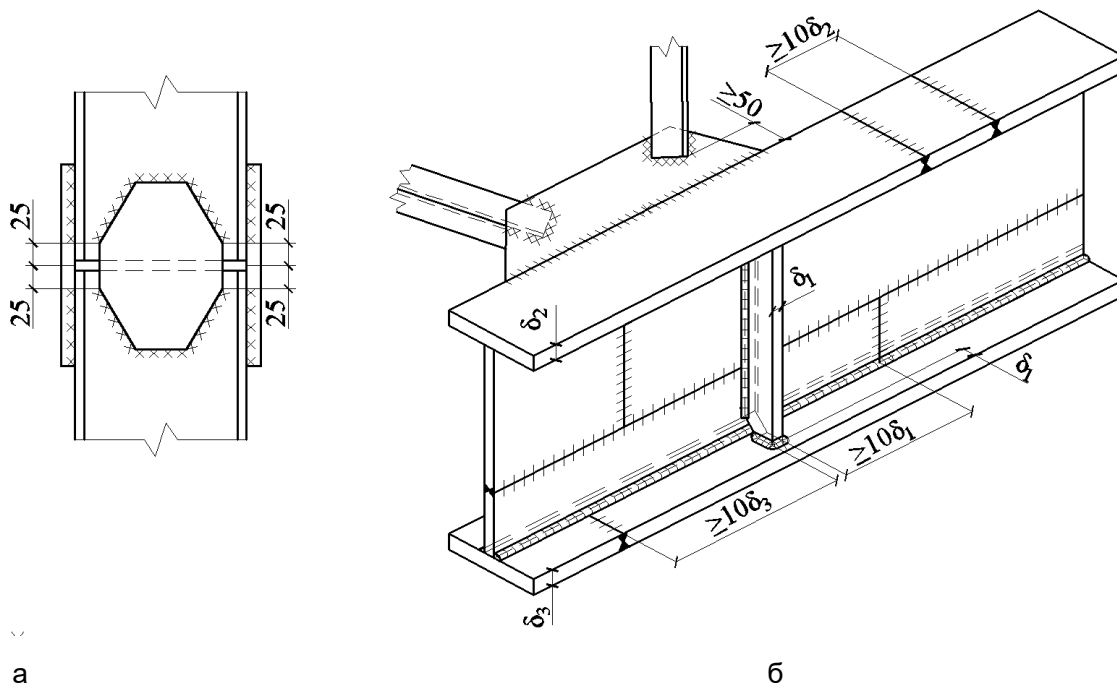
Рисунок 16.2 – Розміщення зварних швів
