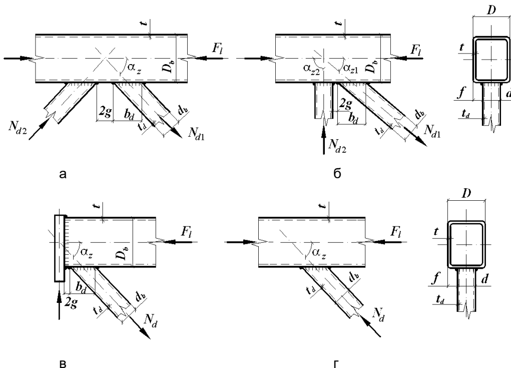
Рисунок Ф.1 – Вузли ферм із гнutoзварних профілів
