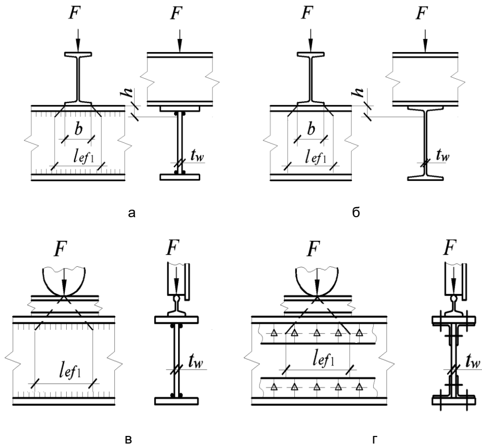
Рисунок 9.1 – Схема передачі зосередженого навантаження на стінку балки
