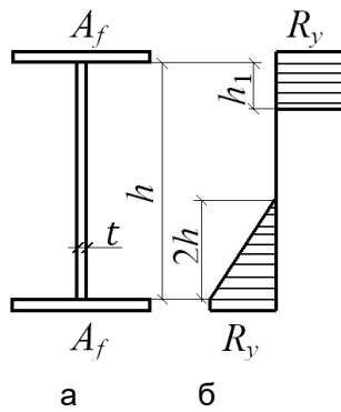
а - переріз балки; б - еюра напружень
