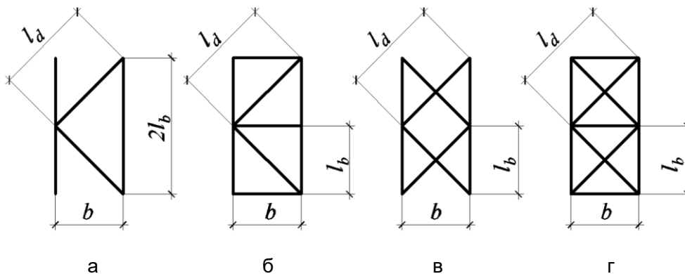
Рисунок 8.2 – Схеми розкісних решіток стрижнів наскрізного перерізу
