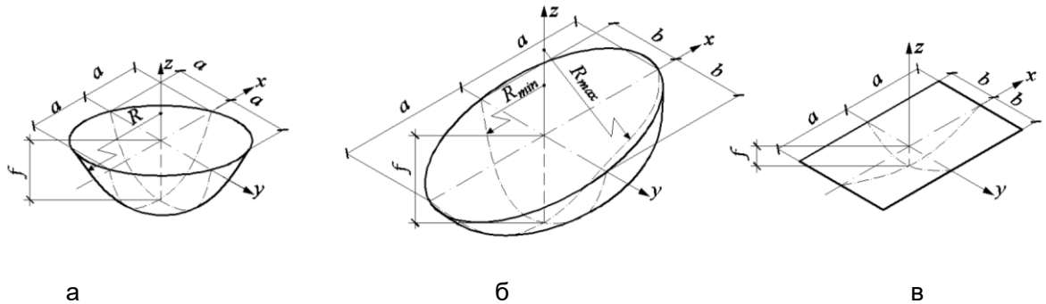
Рисунок 14.4 – Геометрія поверхні оболонки позитивної гаусової кривини
