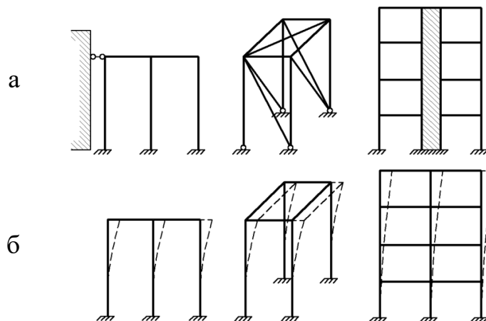
Рисунок 5.2 – Розрахункові моделі несучих конструкцій у вигляді стрижневих систем
