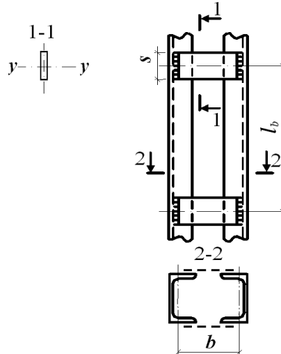
Рисунок 8.3 – Наскрізний стрижень
