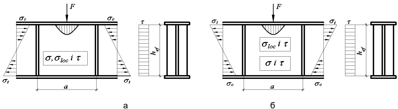
Рисунок 9.3 – Схема ділянки балки, укріпленої поперечними ребрами жорсткості
