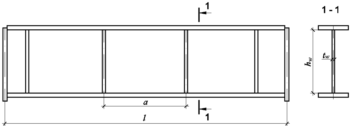
Рисунок 22.1 – Схема балки з гнучкою стінкою
