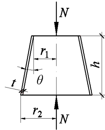
Рисунок 14.3 – Схема конічної оболонки обертання при дії поздовжнього зусилля стиску
