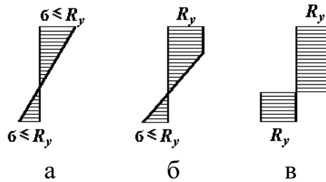
Рисунок 5.1 – Класифікація перерізів за видом НДС
