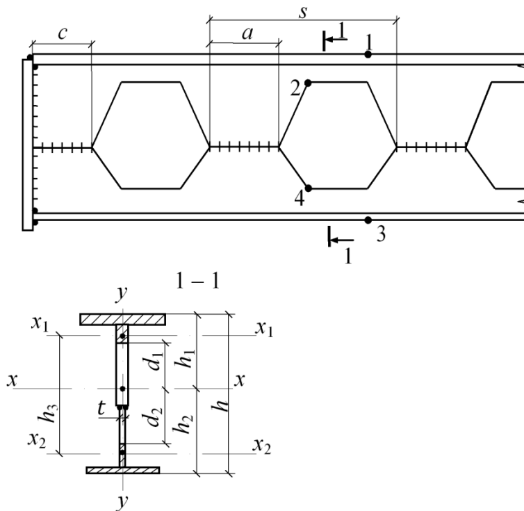
Рисунок 23.1 – Схема ділянки балки з перфорованою стінкою
