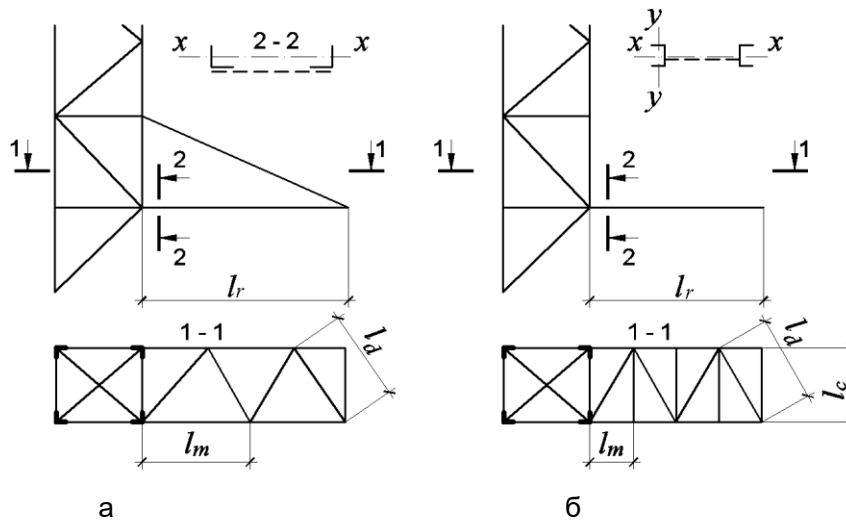
а – з трикутними решітками; б – те саме, зі стояками
