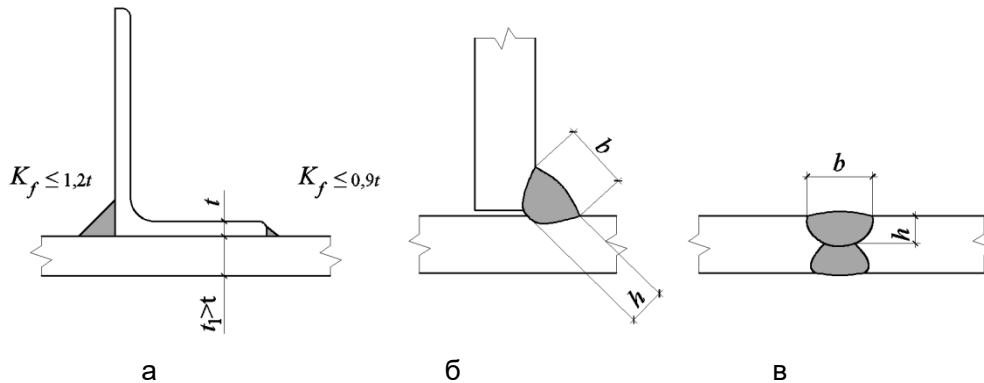
Рисунок 16.1 – Розміри зварних швів
