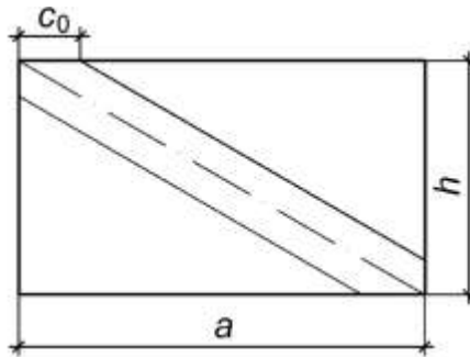
Рисунок Х.2 – Схема відсіку балки при зсуві
