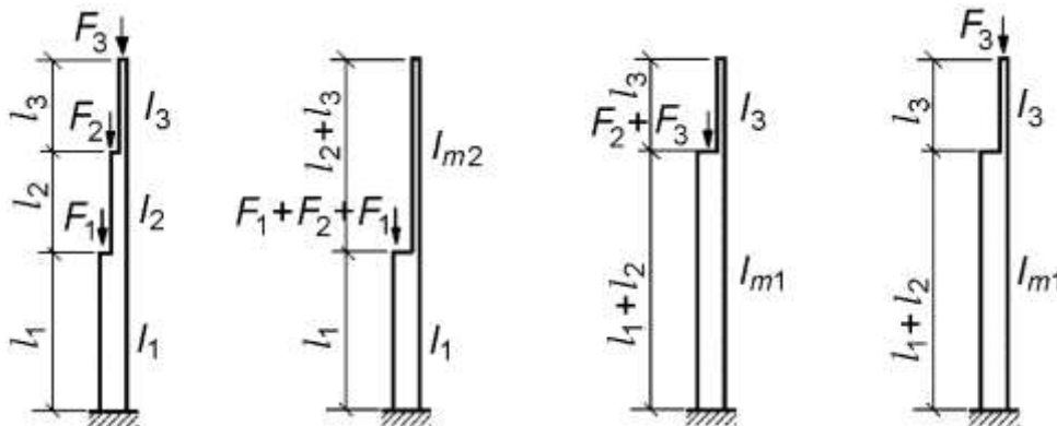
Рисунок С.1 – Схема двоступінчастої колони (а) і умовні схеми навантажень при прикладанні сил F_1, F_2 і F_3 відповідно до верха нижньої (б), середньої (в), верхньої (г) ділянок
