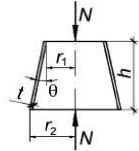
Рисунок 14.3 – Схема конічної оболонки обертанья при дії поздовжнього зусилля стиску
