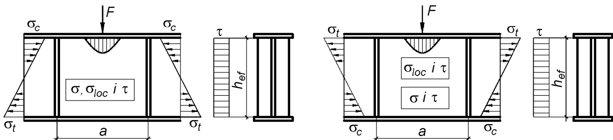
а – при прикладенні зосередженого навантаження до стиснутого пояса; б – те саме до розтягнутого
