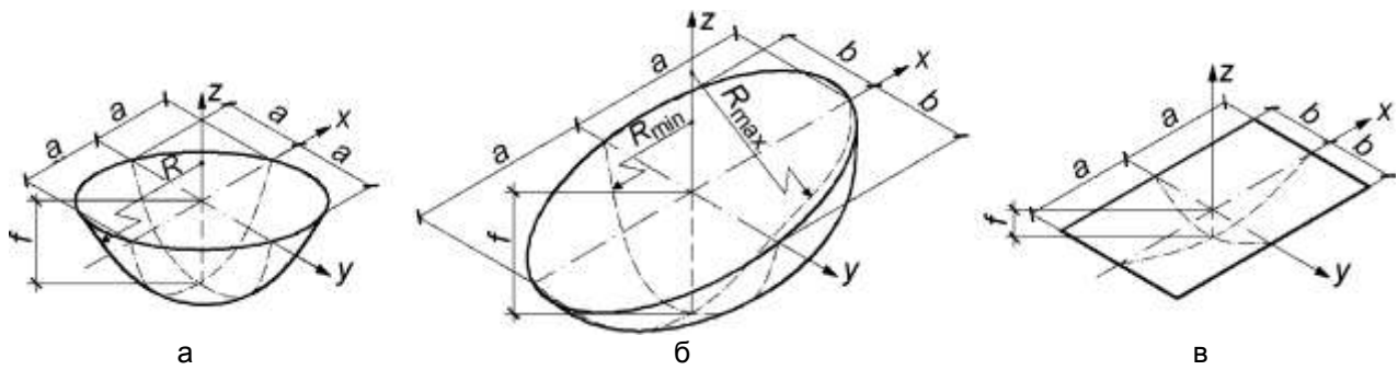
а – на круглому плані; б – на овальному плані; в – на прямокутному плані
