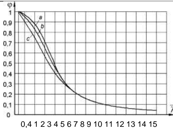
Рисунок Ж.1 – Криві стійкості a, b, c
