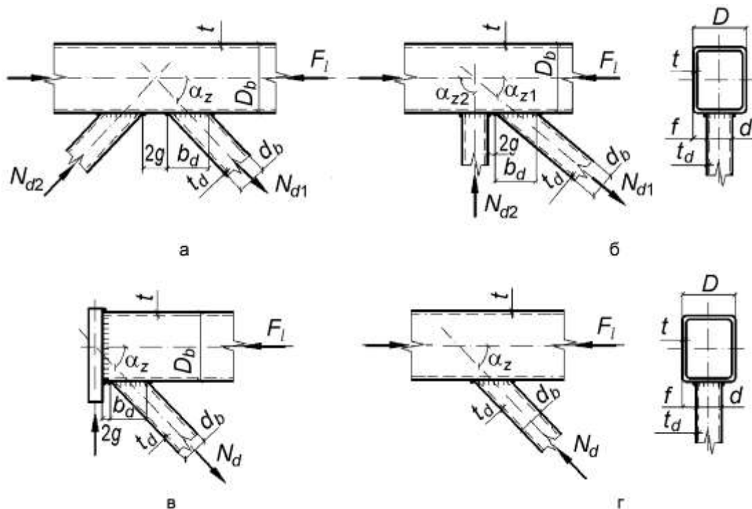
Рисунок Ф.1 – Вузли ферм із гнutoзварних профілів
