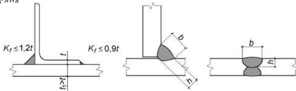
Рисунок 16.1 – Розміри зварних швів
