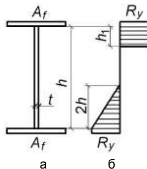
а – переріз балки; б – еюра напружень
