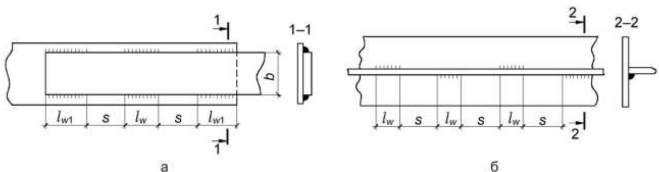
а – у напустковому з'єднанні; б – у тавровому з'єднанні
