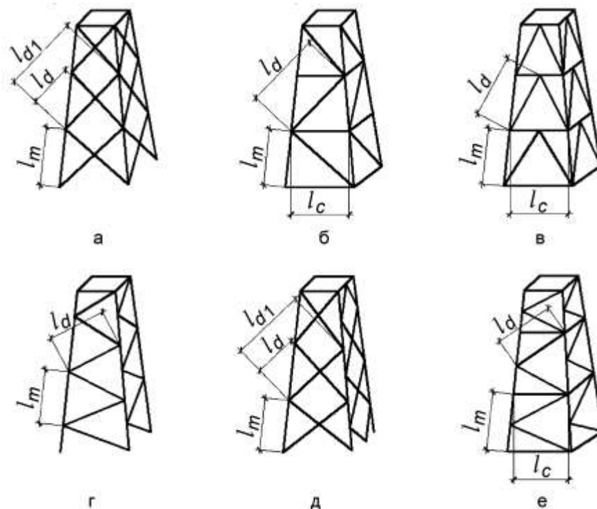
Рисунок 13.3 – Схеми просторових решічастих конструкцій із вузлами в суміжних гранях
