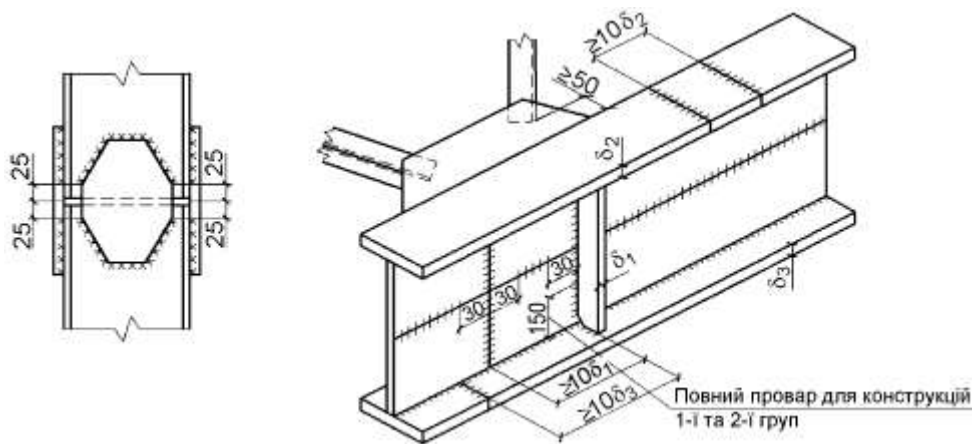
Рисунок 16.1 – Розміри зварних швів
