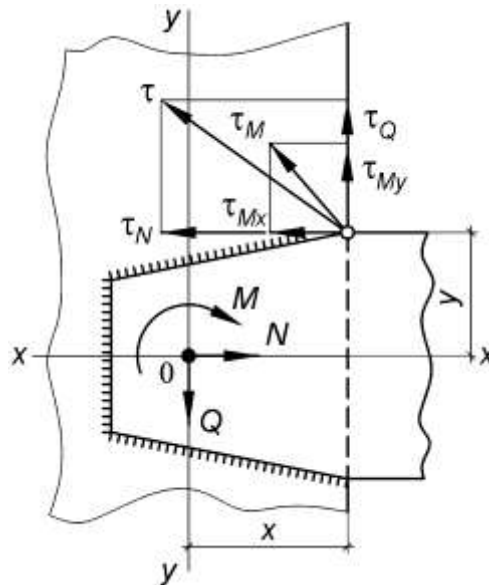
Рисунок 16.5 – Розрахункова схема зварного з'єднання з кутовими швами
