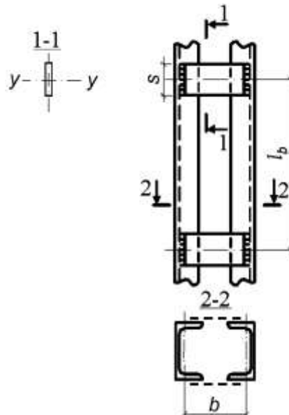
Рисунок 8.3 – Наскрізний стрижень
