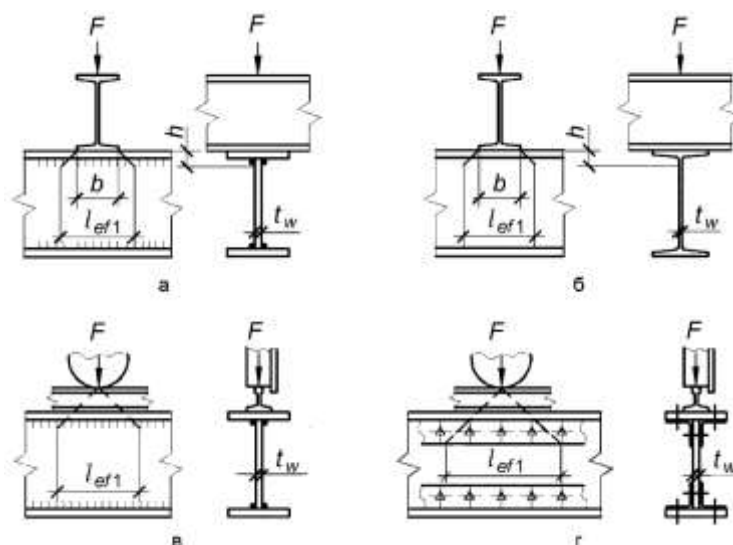
а - зварної; б - прокатної; в - зварної або прокатної від колеса крана; г - з болтовими фрикційними поясними з'єднаннями від колеса крана
