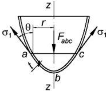
Рисунок 14.1 – Схема оболонки обертанья
