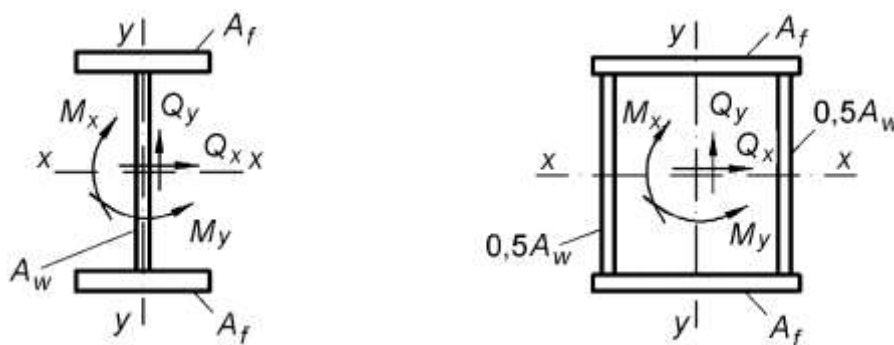
а – двотавровий переріз; б – коробчастий переріз
