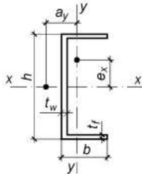
Рисунок К.1 – Схема швелерного перерізу
