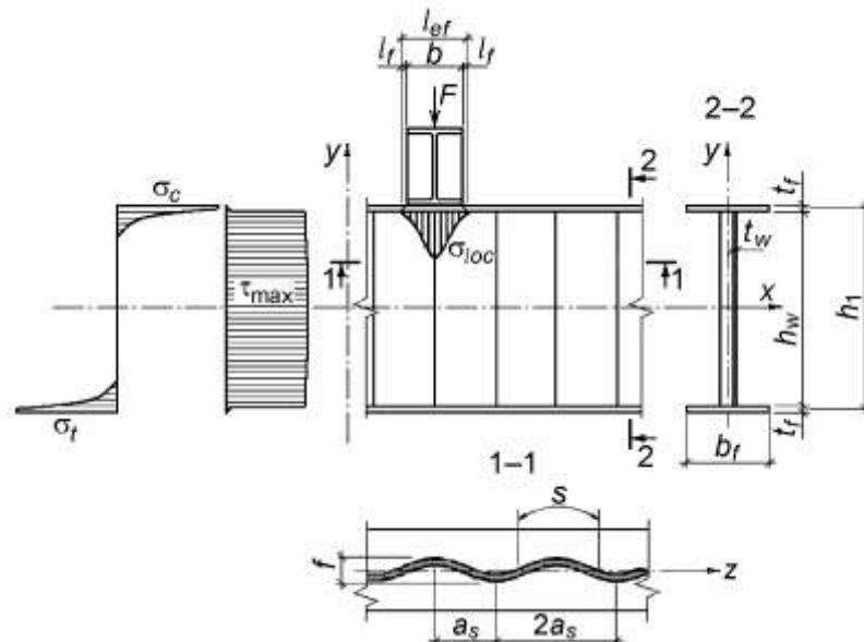
Рисунок 24.1 – Схема елемента з хвилястою (синусоїдною) поперечно гофрованою стінкою
