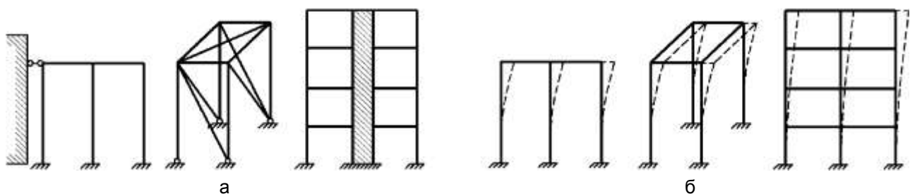
а – системи, закріплені від перекосу; б – системи, не закріплені від перекосу
