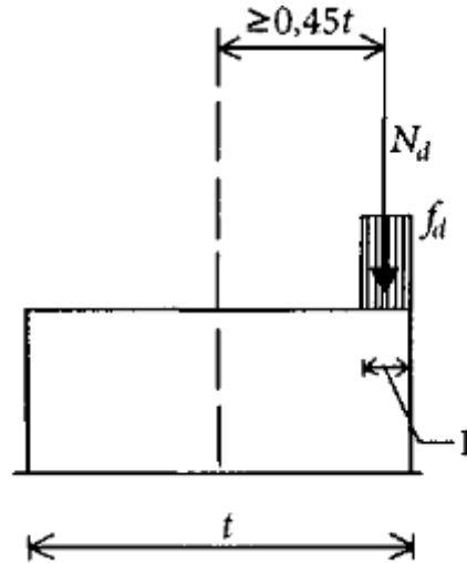
Рисунок В.2 – Ексцентриситет, отриманий за визначенням ділянки опирання, яка необхідна для сприйняття напружень від розрахункового навантаження
