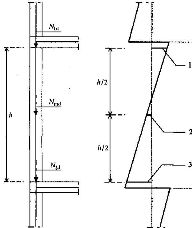
1 – M_{1d} (на нижній стороні перекриття); 2 – M_{md} (на середині висоти стіни); 3 – M_{2d} (зверху перекриття)
