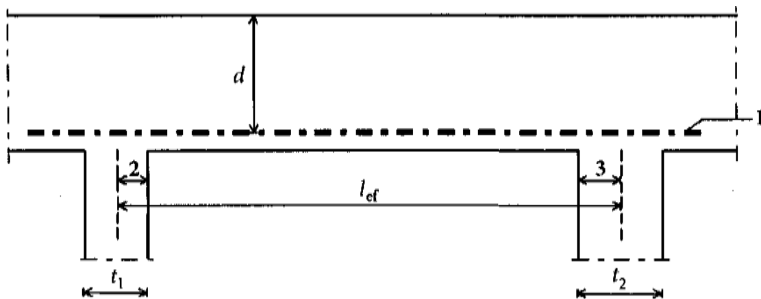
Рисунок 10.3 – Розрахункова довжина прольоту просто закріпленої балки або багатопрольотної балки з кам'яної кладки
