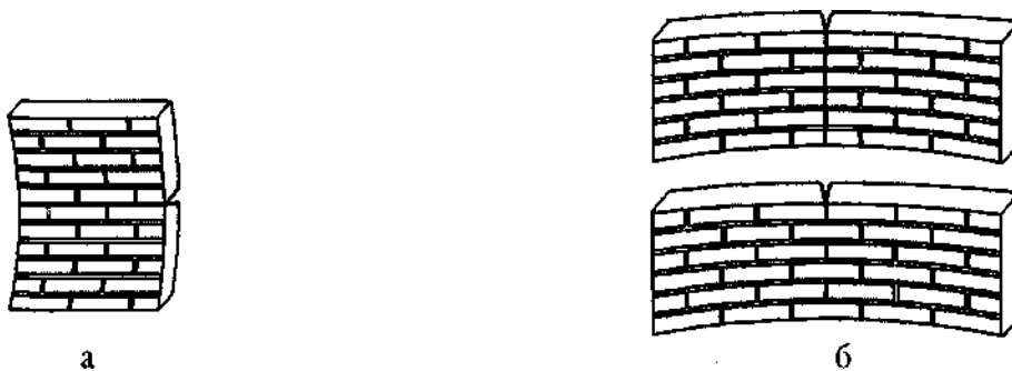
Рисунок 8.1 – Площини руйнування кам'яної кладки при вигині
