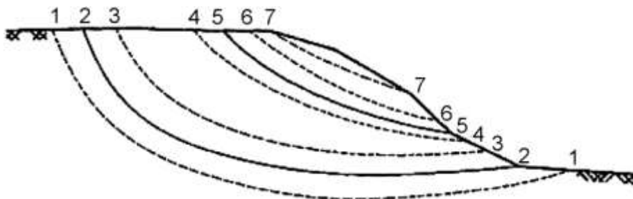
1.7- ймовірні поверхні ковзання
