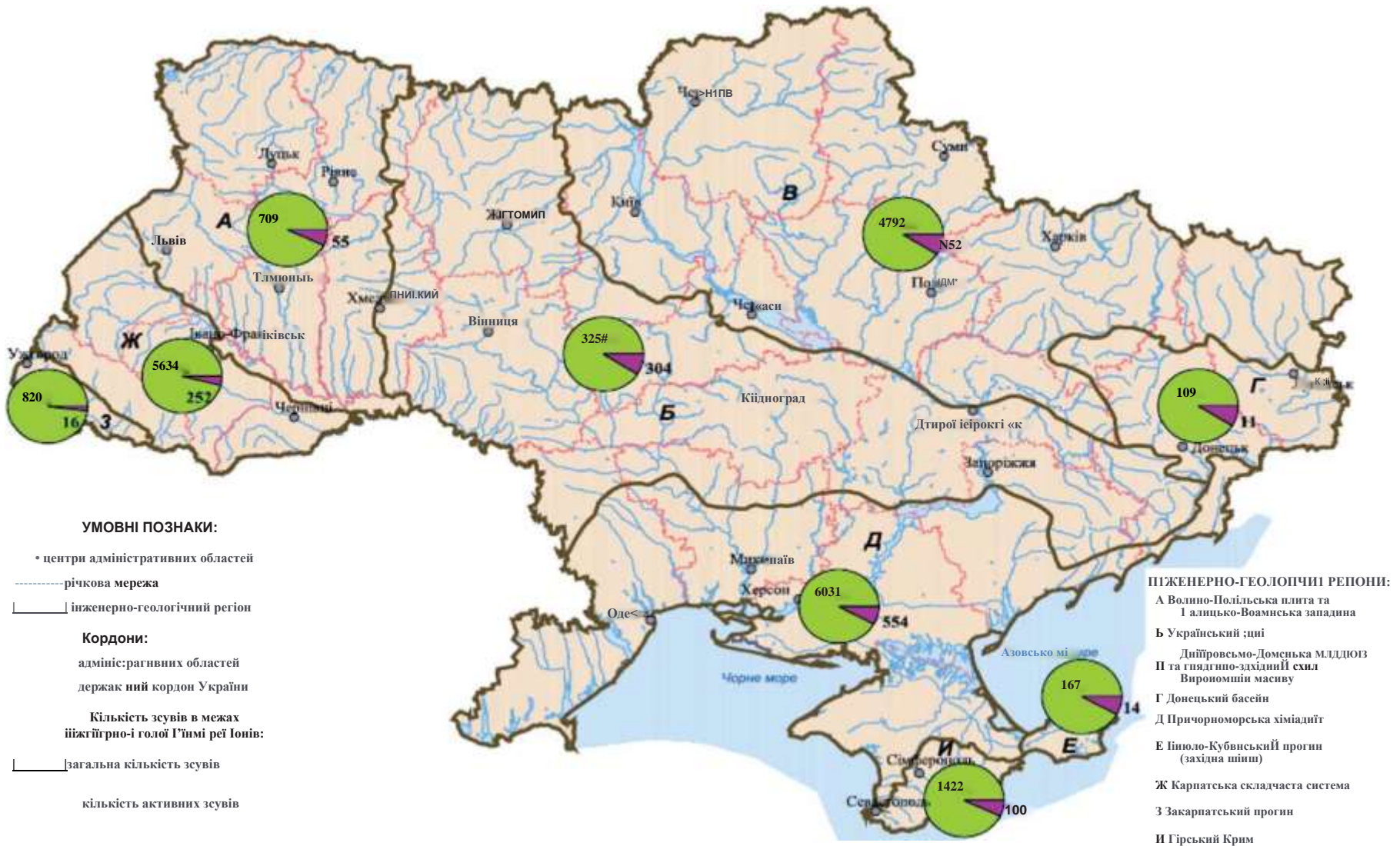
Рисунок А.2 - Поширення зсувів у межах інженерно-геологічних регіонів України
