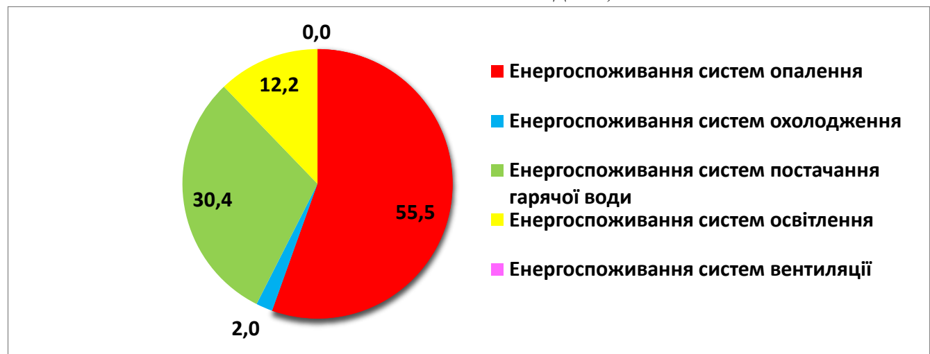
ЕНЕРГОСПОЖИВАННЯ БУДІВЛІ, %
