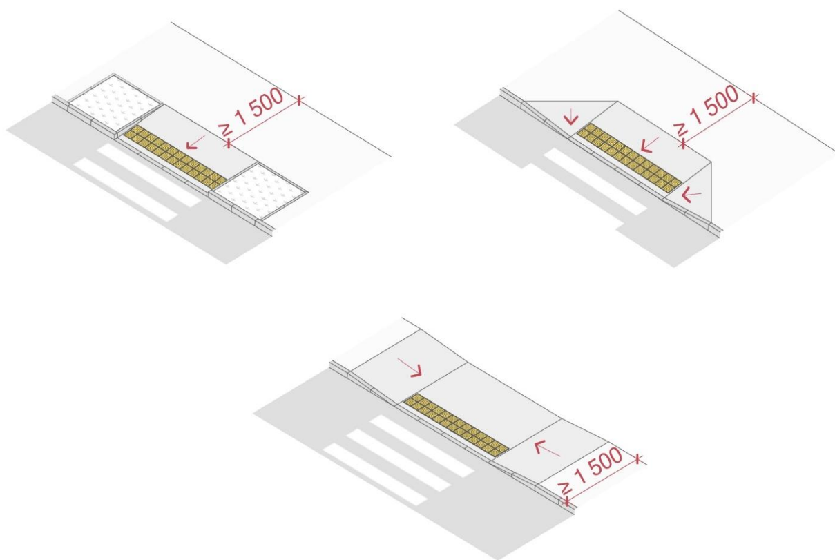
Рисунок 2д — Приклад влаштування бордюрних пандусів
