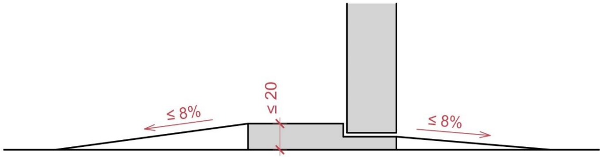
Рисунок 7д — Приклад облаштування дверного порогу (Рисунок 7д додано, Зміна № 3)
