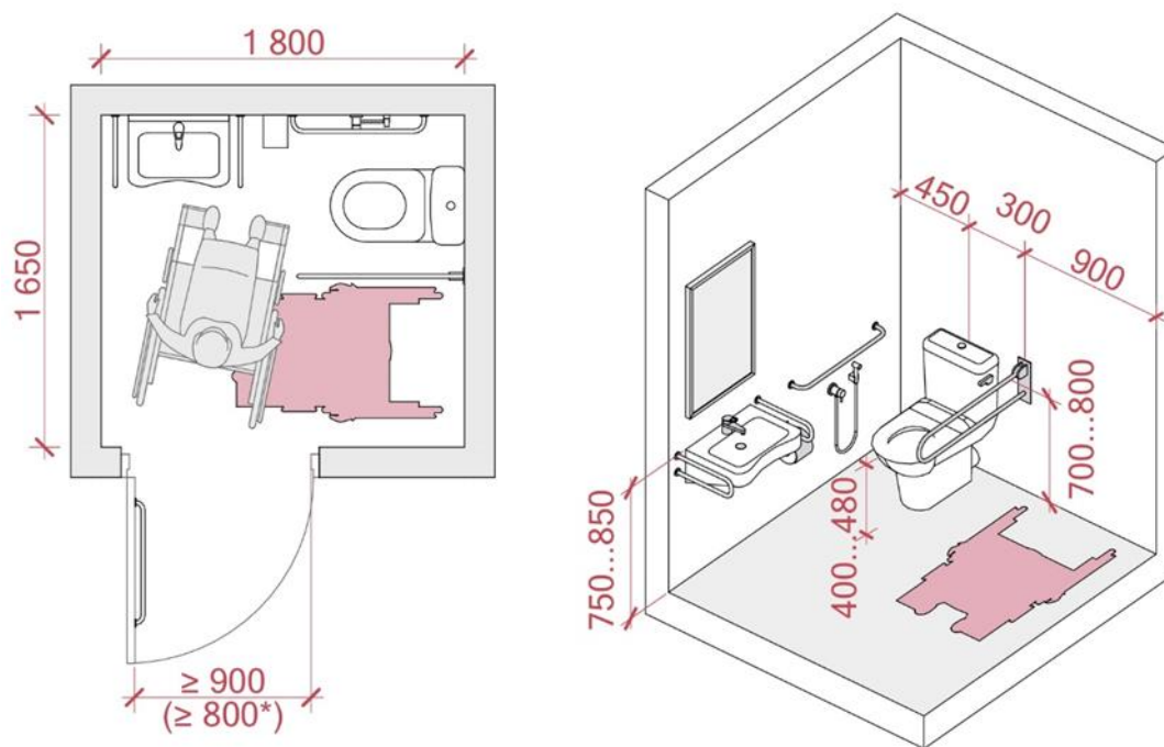
Рисунок 42 — Приклад облаштування та розміщення обладнання універсального санітарно-гігієнічного приміщення (універсальної кабінки туалету загального користування) при реконструкції та капітальному ремонті
