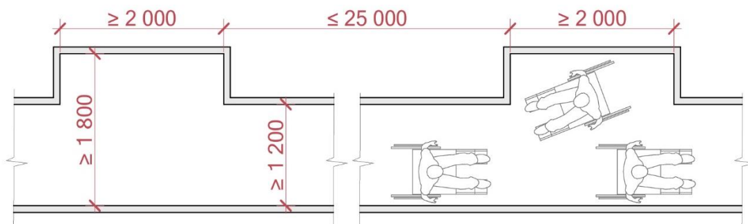
Рисунок 1в — Приклад влаштування пішохідної доріжки з роз'їзними кинями
