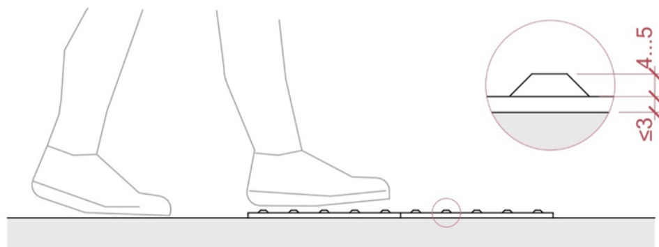
Рисунок 28б — Приклад укладання тактильного індикатора на поверхні шляху руху
