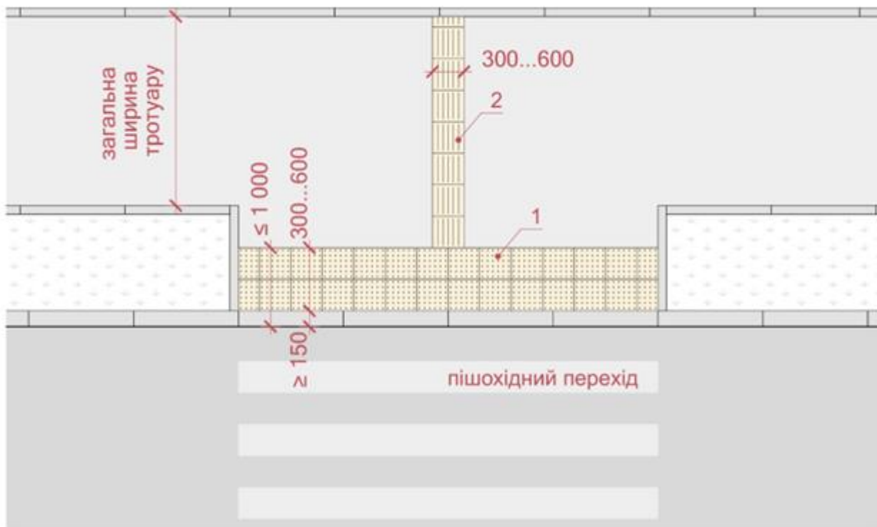
Рисунок 33а — Застосування спеціальних ТС на наземних пішохідних переходах
