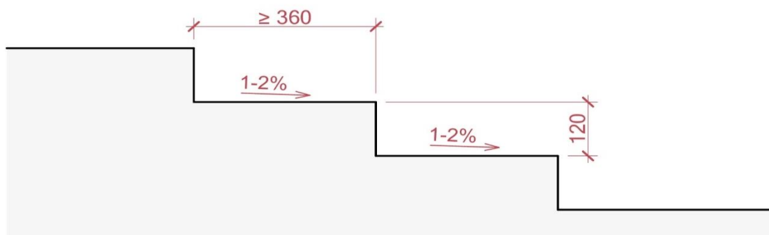
Рисунок 46 — Параметри відкритих сходів та ґанків
