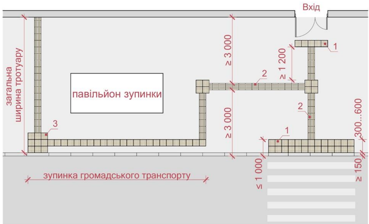
Рисунок 32а — Приклад улаштування маршруту руху за допомогою системи спеціальних ТС від входу/виходу з будівлі до основних об'єктів дорожнього простору
