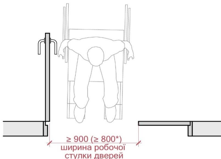
Рисунок 7е – Ширина робочої частини (стулки) в просвіті
