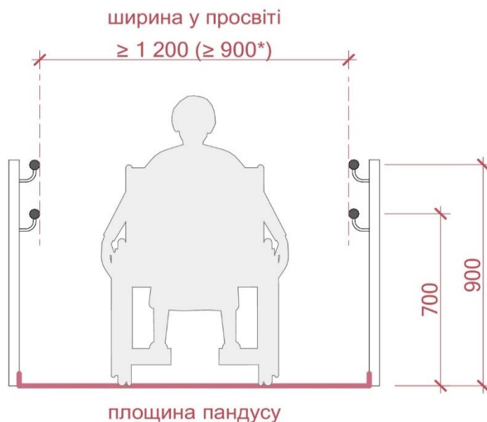
Рисунок 5д — Ширина пандуса у просвіті
