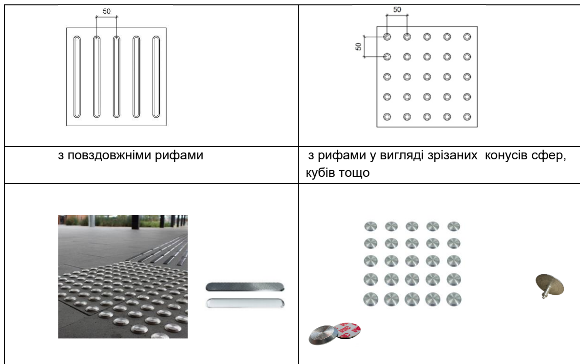
Рисунок 28а — Спеціальні тактильні індикатори
