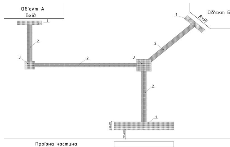
Рисунок 31а — Приклад улаштування маршруту руху за допомогою напрямлюючої ТС від входу/виходу з будівлі до основних об'єктів дорожнього простору:
