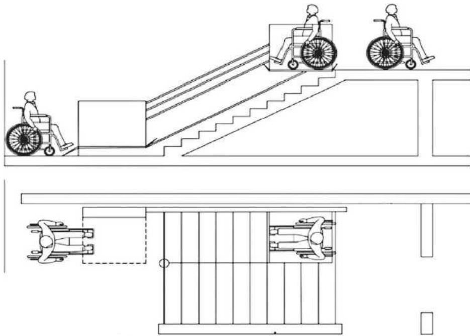
Рисунок 12 - Індивідуальні підйомники (похилі).
