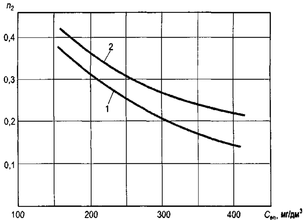
Рисунок В.1 – Залежність показника ступеня n_2 від концентрації завислих речовин C_{en} у міських стічних водах при ефекті освітлення 50 % та 60 %
