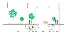
Проектируемый поперечный профиль №- (ул. Школьная)
