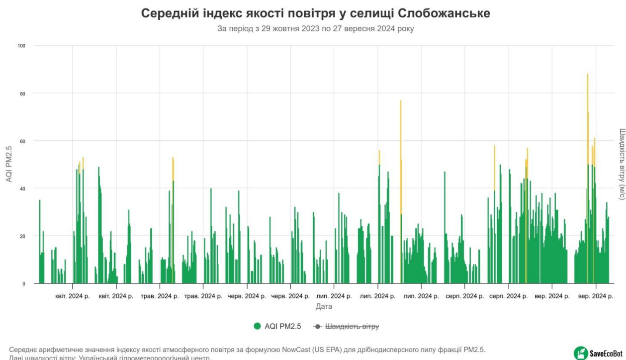
Рисунок 3.8 – Середнє арифметичне значення індексу якості атмосферного повітря
