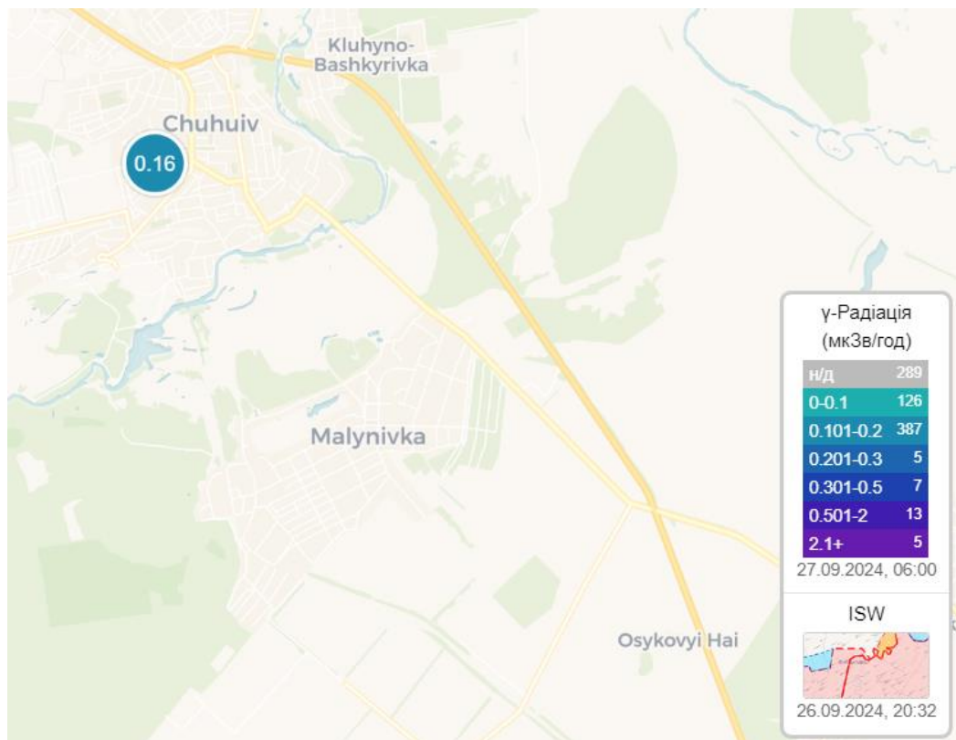
Рисунок 3.9 – Радіаційний фон м. Чугуїв (станом на 27.09.2024)
