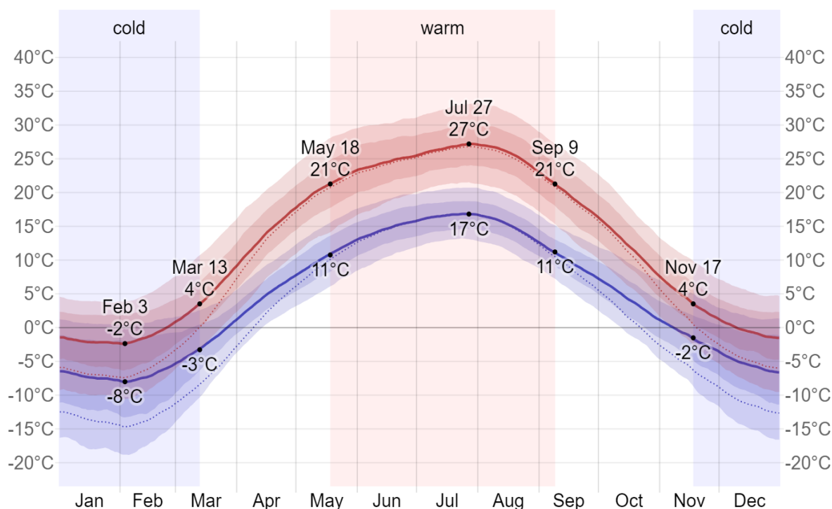
Рисунок 3.1 – Середня максимальна і низька температура в м. Чугуїв 6
