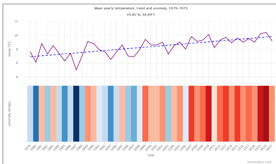
Рисунок 3.2 – Середньорічна зміна температури для міста Чугуїв, тенденція та аномалія, 1979 – 2023 роки 7
