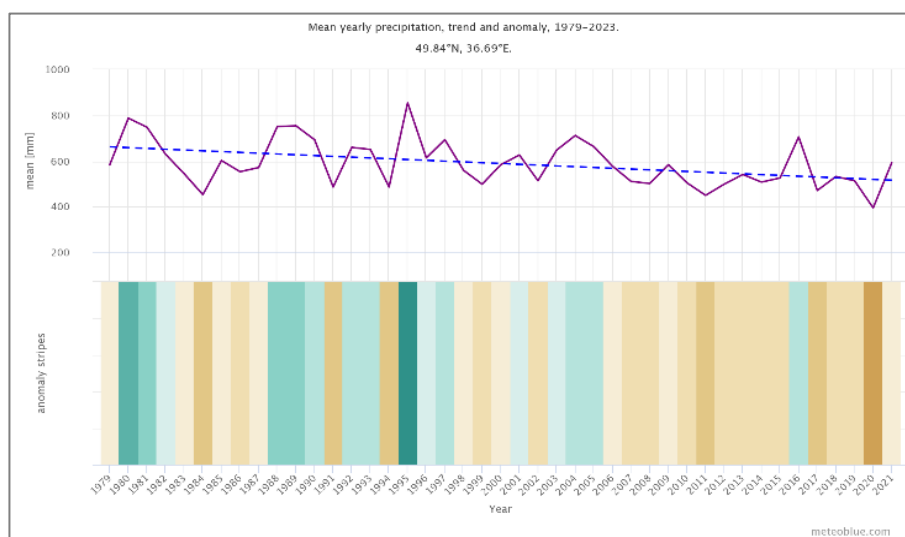
Рисунок 3.3 – Середньорічна кількість атмосферних опадів для міста Чугуїв, тенденція і аномалії, 1979 – 2023 роки 8
