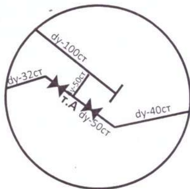
Колодязь ВК-1
