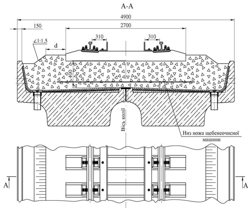
Рисунок Г.1 – Мостове полотно з їздом на щебеневому баласті і залізобетонних шпалах з роздільними клебно-болтовими рейковими скріпленнями з різьбовим прикріпленням рейки і підкладки до шпали
