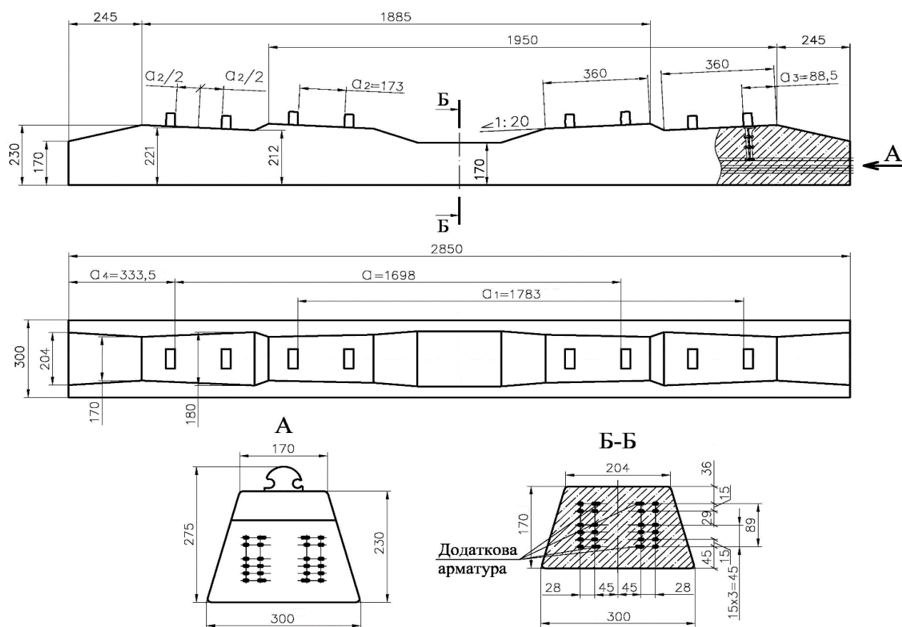
Рисунок В.5 – Шпала залізобетонна суміщеної колії 1520 мм і 1435 мм з рейками типу Р65 або UIC60 (60Е1) і безпідкладковим анкерним пружним рейковим скріпленням з безрізьбовим прикріпленням рейки до шпали
