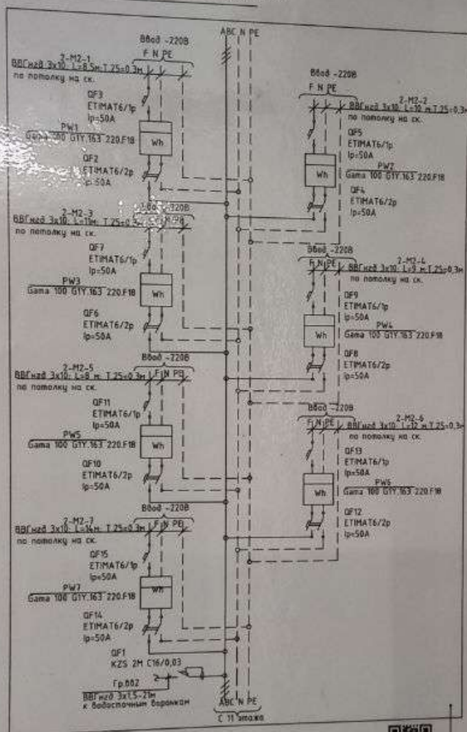
Однолинейная принципиальная схема щита этажного 2.10(3.12)
