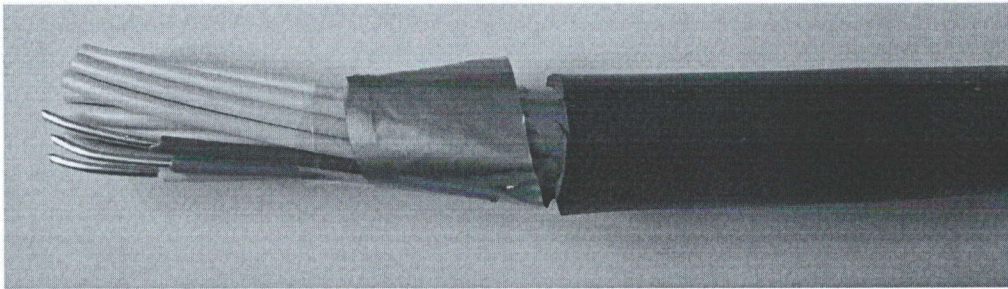
Рис. 1 — Конструкція зразка кабелю КВВГЕнг-LS 27х2,5.
