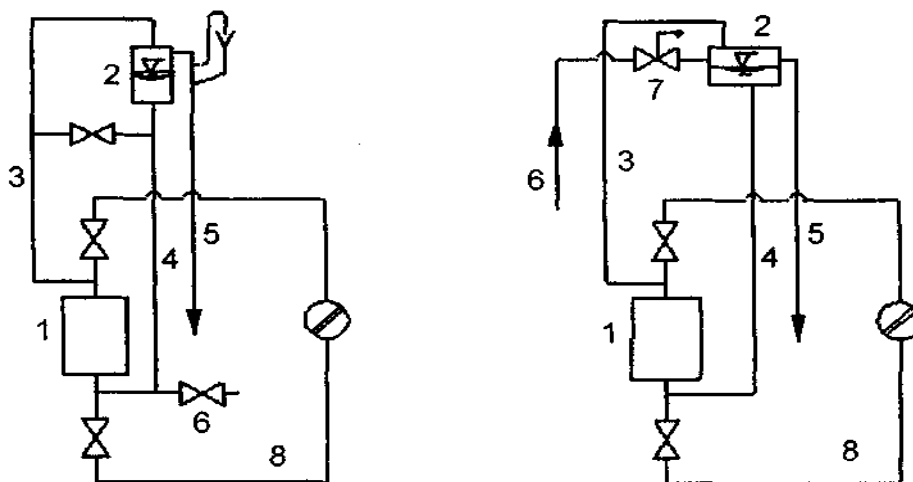
1 - теплогенератор; 2 - розширювальний бак; 3 - запобіжний трубопровід; 4 - з'єднувальний трубопровід; 5 - переливний трубопровід; 6 - трубопровід для заповнення системи; 7 - обмежувач рівня води; 8 - зворотний трубопровід
