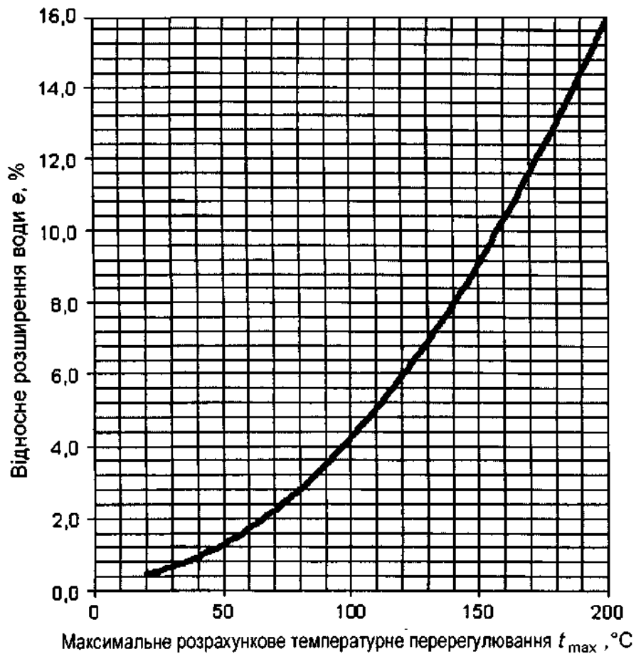
Рисунок Л.2 - Графічна залежність відносного розширення води від максимального розрахункового температурного перегріву за температури заповнення 10 °C
