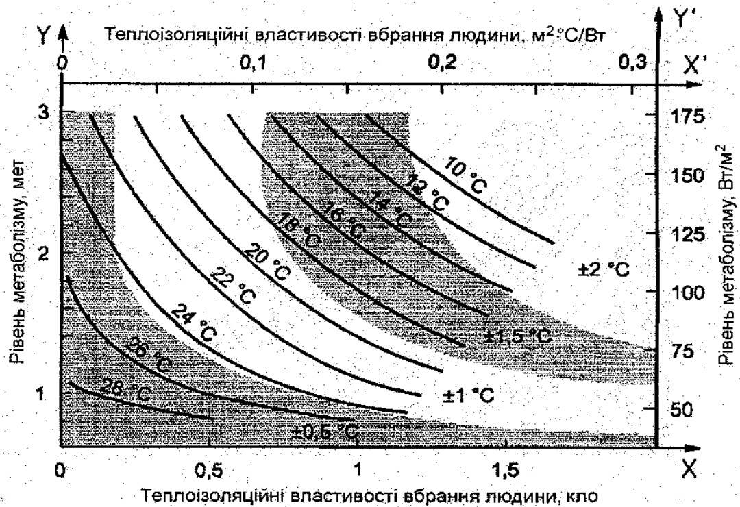
Рисунок Д.1 – Результуюча температура та її допустимий діапазон підвищених оптимальних умов мікроклімату приміщення
